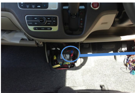
シフト+エアコンパネルカバー裏のハザードスイッチカプラ
