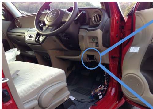
運転席右寄り足元のヒューズボックス
